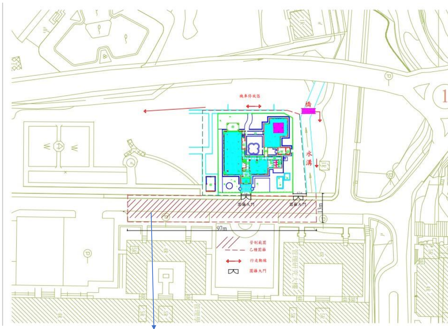
蔣介石行館鋼棚架拆除封閉-施工範圍平面圖
